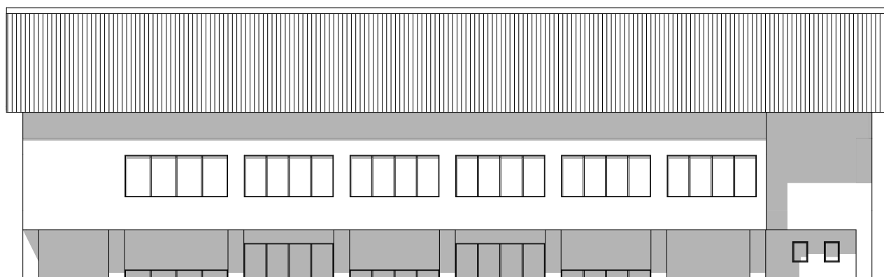
西側立面図
