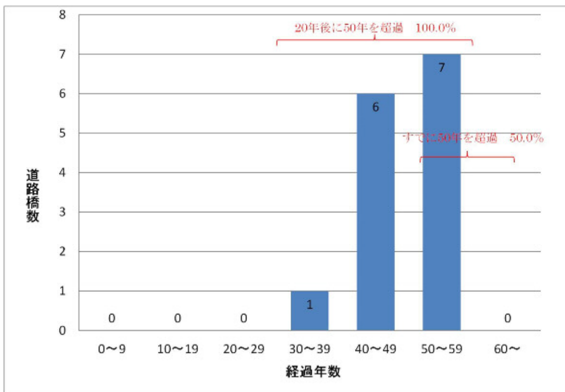
図2-1 本計画の対象とする林道橋の経過年数ごとの橋梁数
